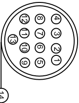
FRONT VIEW 13PIN DIN JACK
